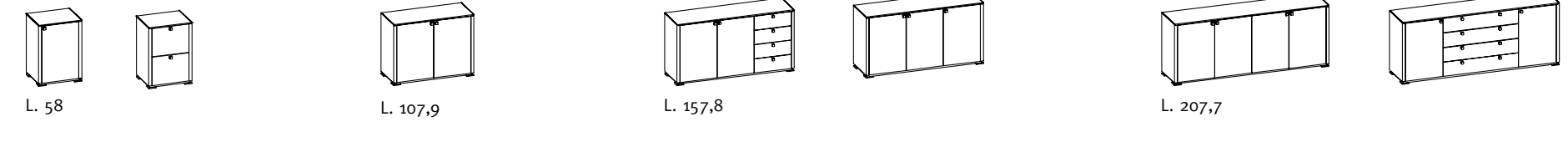
L. 58 L. 107,9 L. 157,8 L. 207,7
