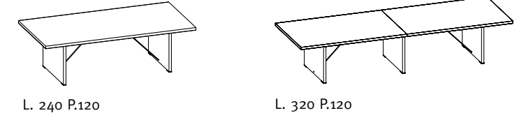
L. 240 P.120 L. 320 P.120
